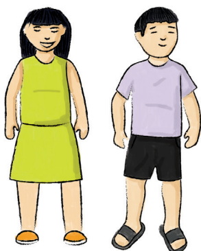
2- Ni
